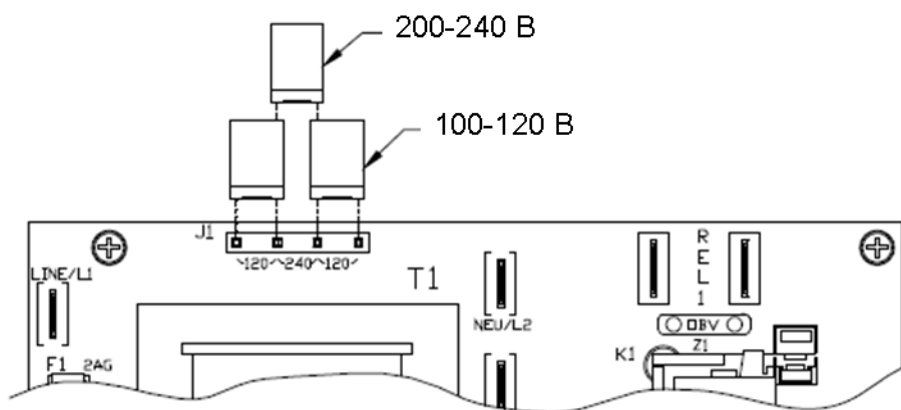
Рис. 2. Переключающая колодка.
