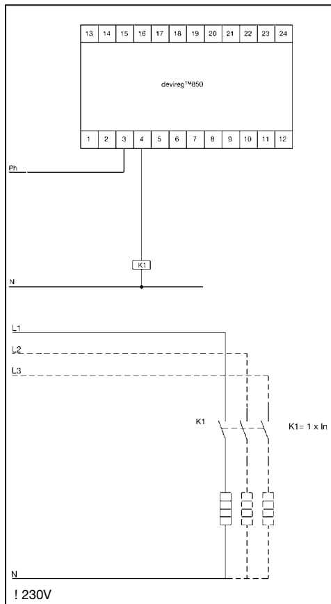
Рис. D. Крылья, 1-3 фазы, 1-3 кабеля на 230
